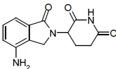
3-(7-amino-3-oxo-1H-isoindol-2-yl)piperidine-2,6-dione
